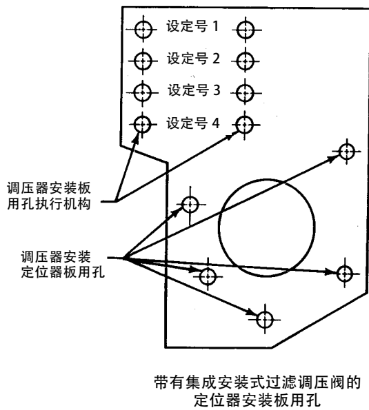
图 5. Fisher 3582 阀门定位器的安装板
