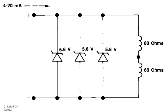
图 10. Fisher 582i 型转换器的输入等效电路
