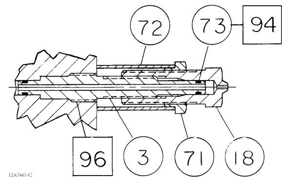
图 21. 喷嘴部件
