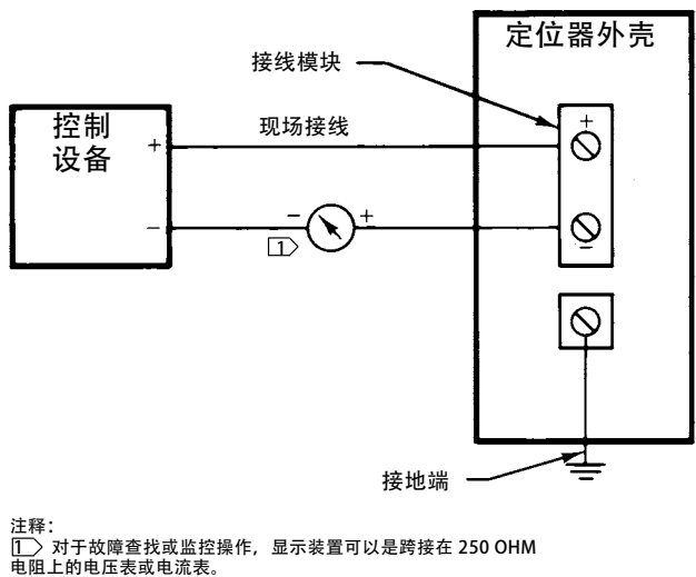
图 9. 典型现场接线图
