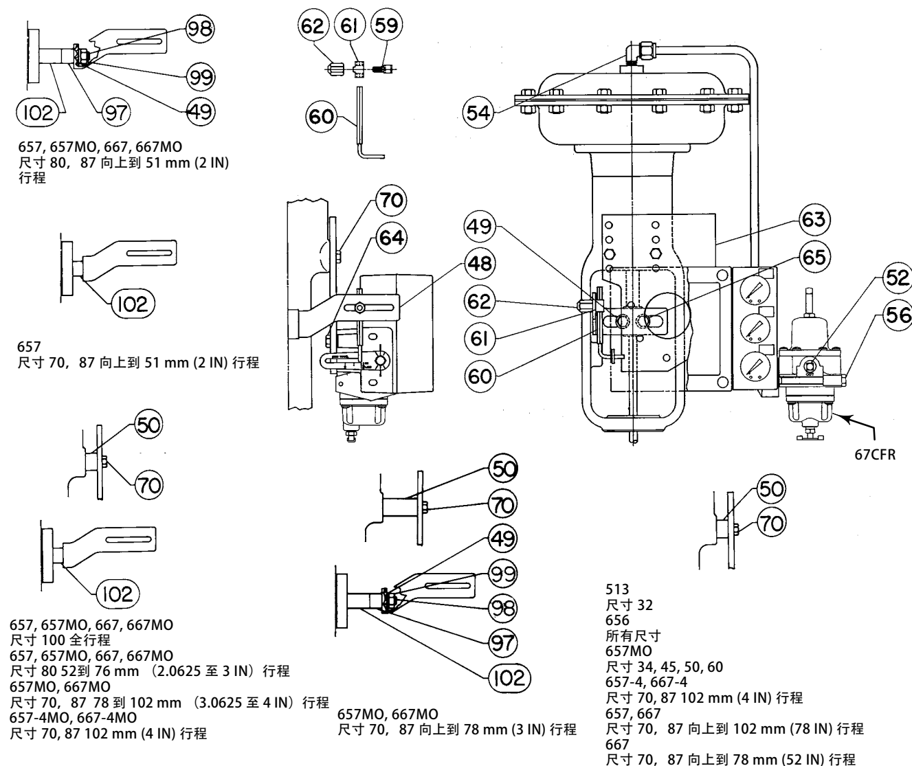
图 2. 安装组件
