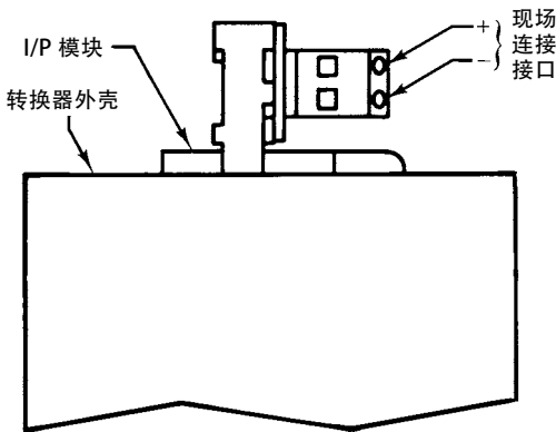
图 11. Fisher 582i 型转换器的导线连接
