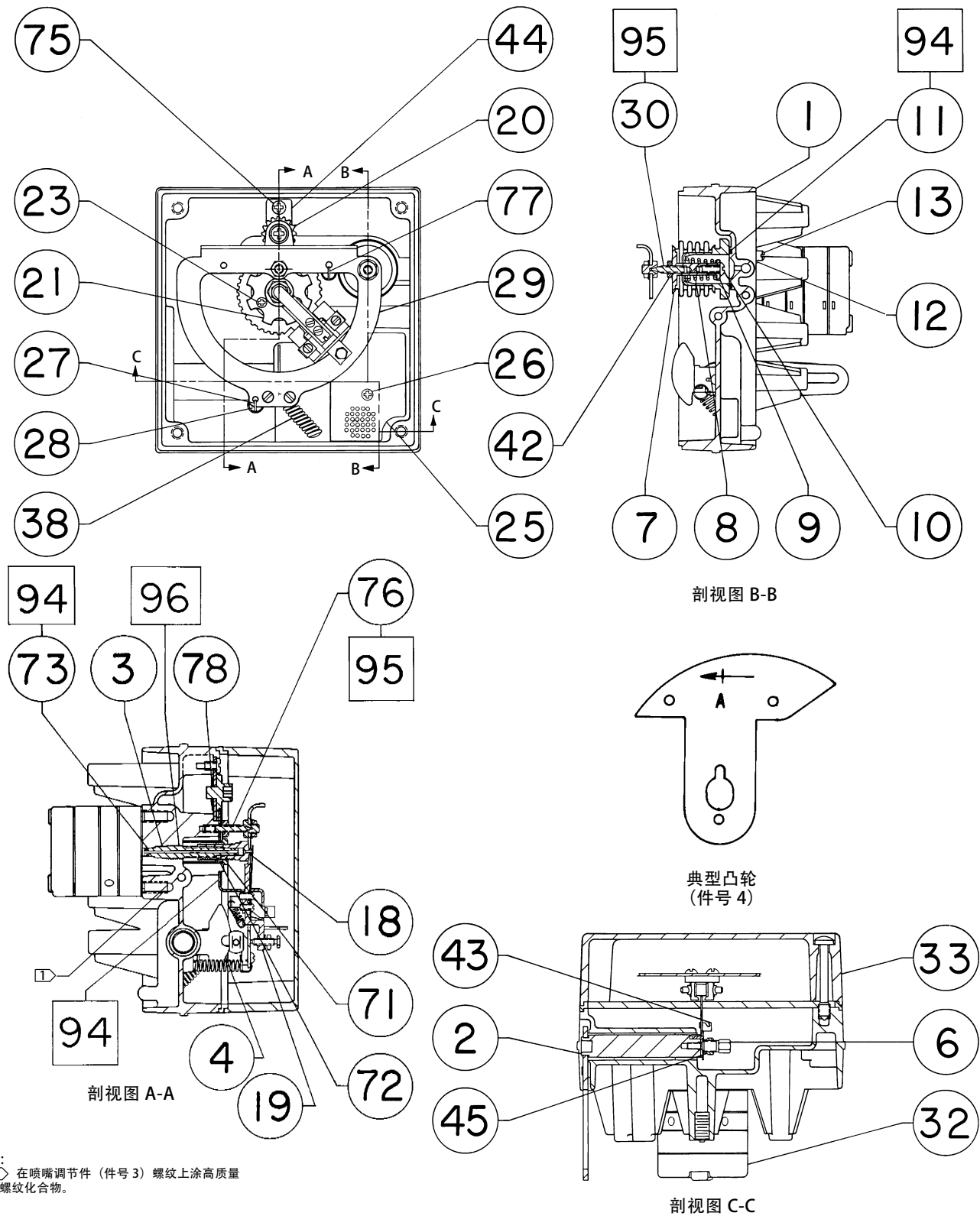
图 20. Fisher 3582 型定位器装配图
