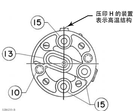
图 22. 83L 放大器
