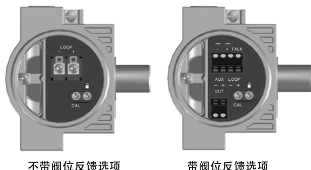
图 7 - 1. 接线盒
