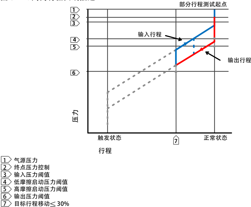
图 3 - 4. 阀门特性曲线描述
