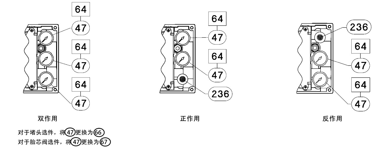
图 7 - 3. 压力表配置
