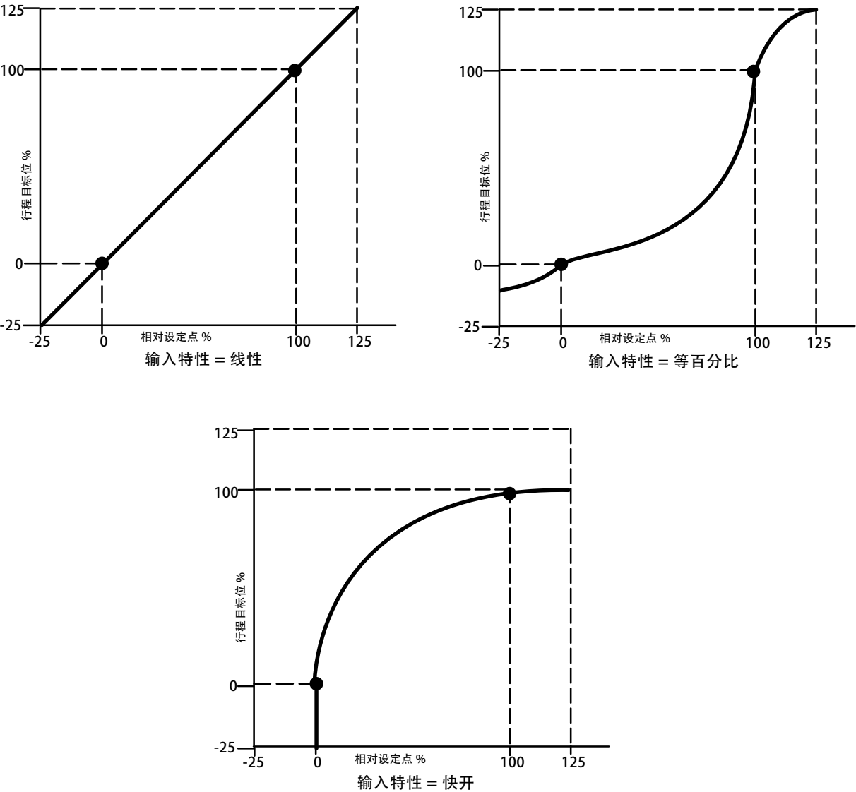
图 3 - 2. 各种输入特性的行程目标位与相对设定点之间的关系曲线（零功率状态 = 关闭）
