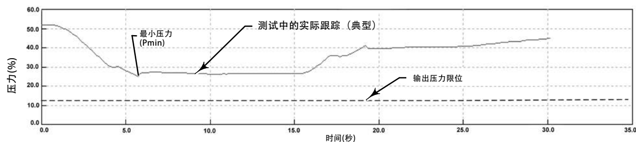
图 3 - 6. 时间序列细节示例；执行机构压力
