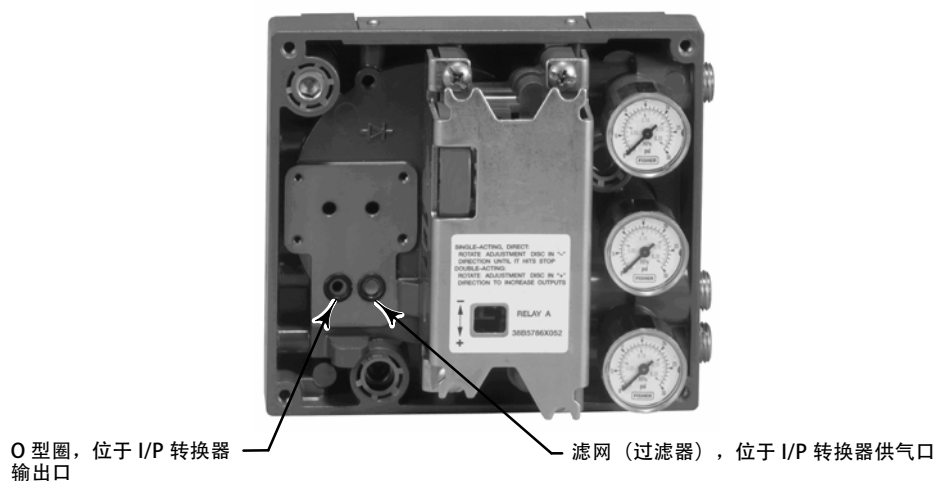
图 6-2. I/P 过滤器的位置
